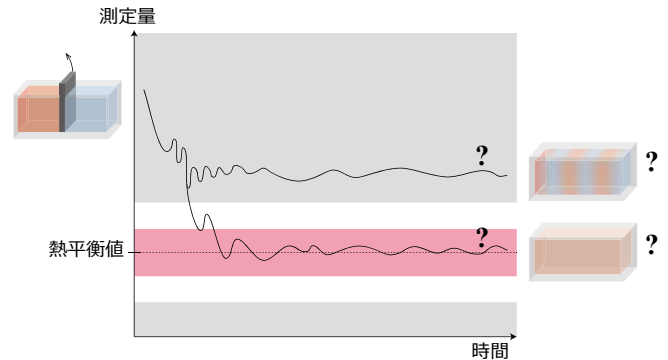
図1 孤立量子系の熱平衡化の問題状況。
