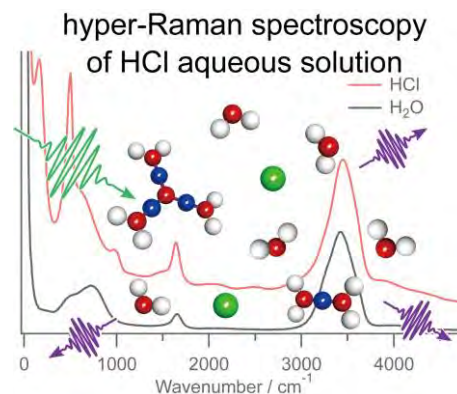
図3 塩酸のハイパーラマン分光&ハイパーラマンスペクトル
