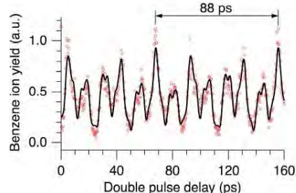
高強度レーザー光を照射したベンゼンの励起スペクトル（上） ポンプ-プローブ法によるベンゼンの回転運動の追跡（下）
