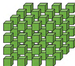
図2. テンソルデータ (三次) の例。数を三次元空間に並べた形で、ベクトルのテンソル積で定義される。
