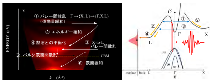
角度時間分解2光子光電子分光によるGeのバレー間散乱の観測。(大阪市大との共同研究)
