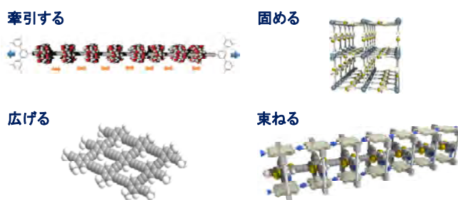
分子建築学による高分子共役鎖の熱的ゆらぎ抑制
